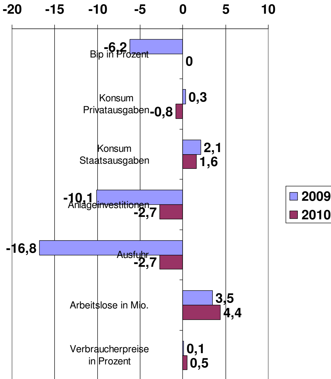
Abbildung 1 Bundesbankprognose vom 04.06.2009
